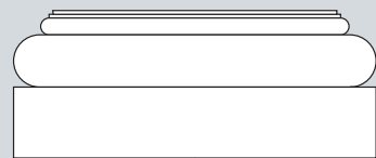
BSE 18-T • 24" square x 9 7/8" h. • To fit CLM 1813-SM
